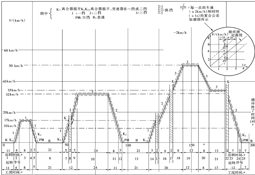
图 C.1 瞬态工况运转循环
